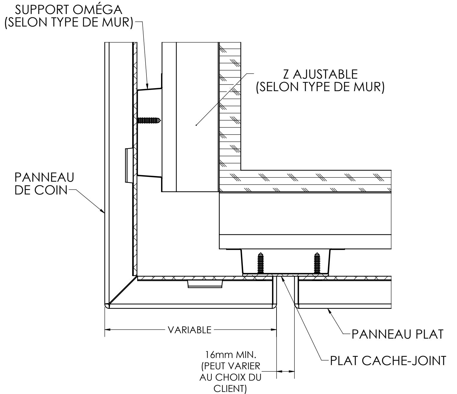
DÉTAILS COIN EXTÉRIEUR AVEC PANNEAU DE COIN (VUE EN PLAN)
