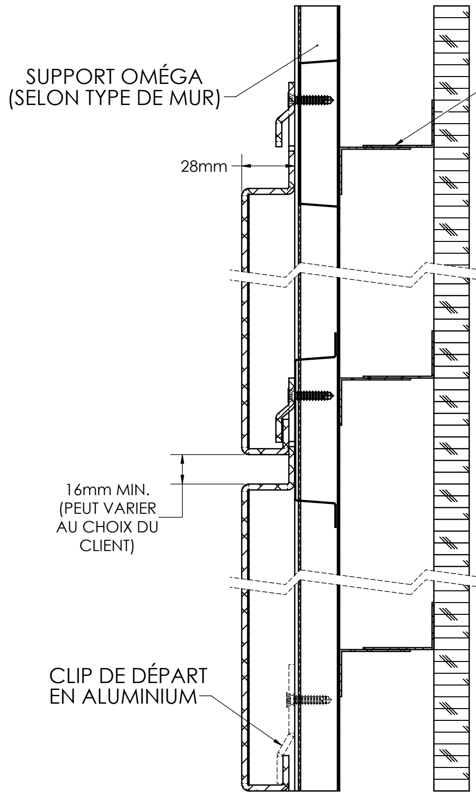
DÉTAILS D'ASSEMBLAGE (VUE EN ÉLEVATION)
